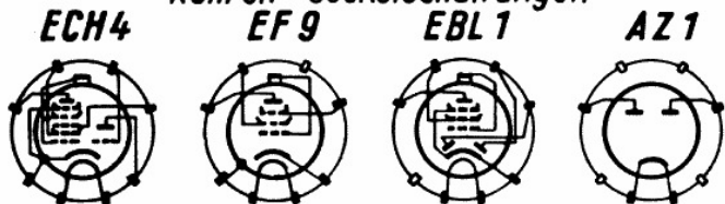
Anschlüsse von unten gesehen
